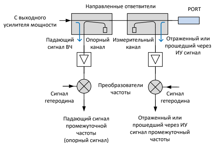
Рисунок 2.5 Группа выделения и преобразования сигналов
