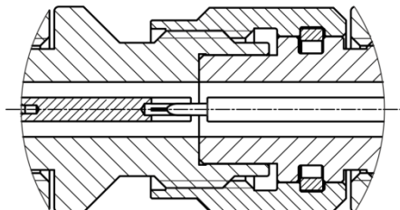
Рисунок А.3 Пример подключения Соединители 1,85 мм (розетка слева, вилка справа)
