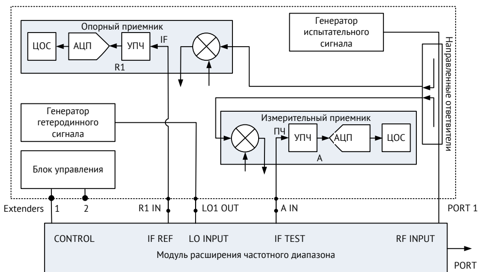
Рисунок 2.9 Схема подключения модуля к анализатору
