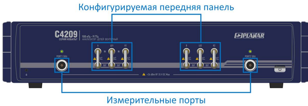
Рисунок 4.3 Передняя панель
